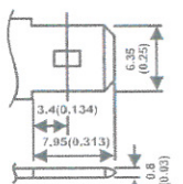
F2 (Faston Tab 250)
